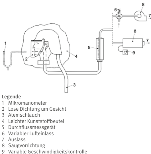
Abb. 28 Typische Anordnung zum Prüfen der Volumenströme der Luftversorgung bei Hauben mit lose sitzender Halsabdichtung
