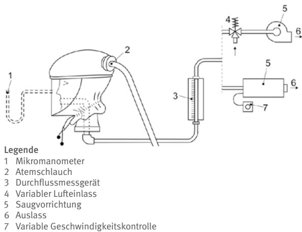
Abb. 27 Typische Anordnung zum Prüfen der Volumenströme der Luftversorgung bei Hauben mit dicht sitzender Halsabdichtung
